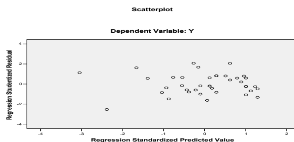
Gambar 1. Uji Heteroskedastisitas
